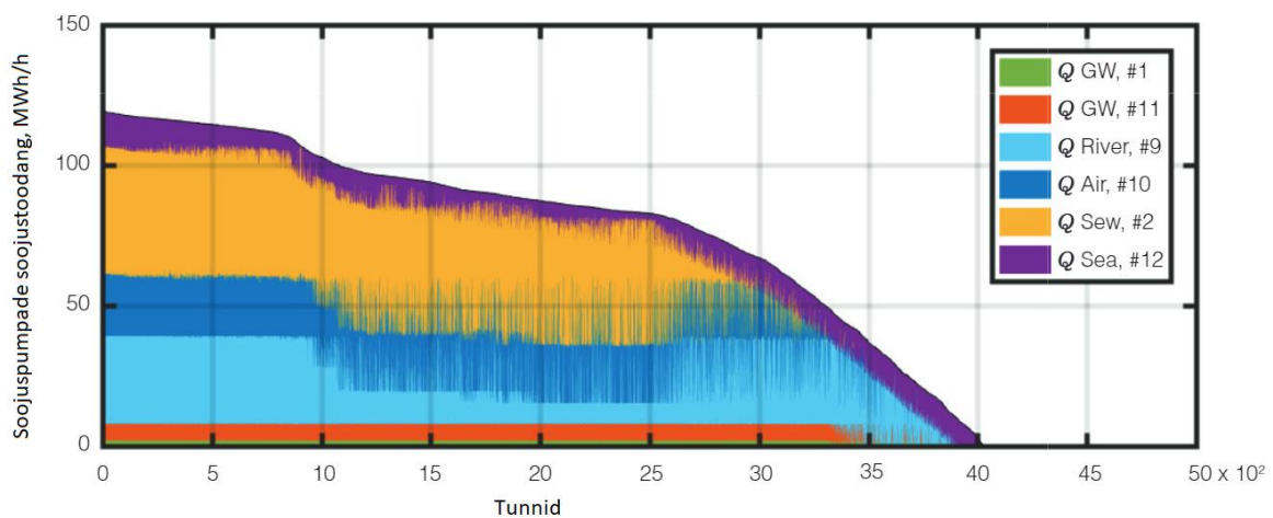
Joonis 10.12. Soojuspumpade koormuse kestuskõver
