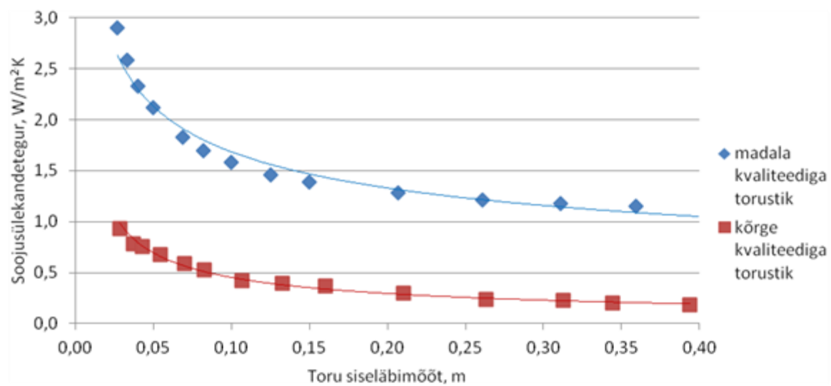
Joonis 5.2. Üldine soojusülekanndetegur kõrge kvaliteediga uutel torudel (eelisoleeritud) ja vanadel torudel (betoonkünades mineraalvillaga isoleeritud torud)
