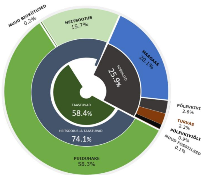
Joonis 1.11. Toodetud soojuse jaotus selle tootmiseks kasutatud kütuse/energia järgi kaugküte sektoris (allikas: Eesti kaugküte sektori CO 2 heitmed, 2021)
