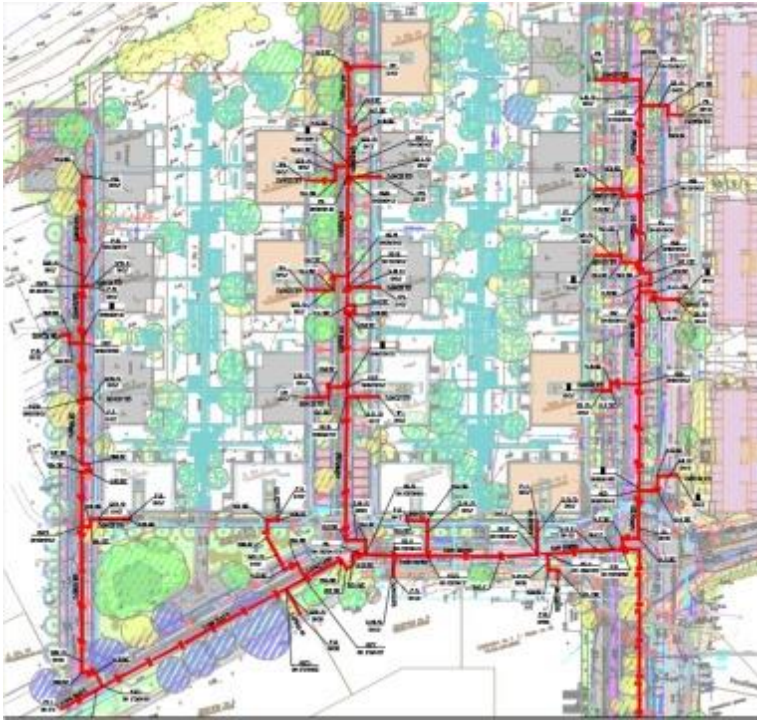
Joonis 10.3. Kopli liinidel arendatava piirkonna skemaatiline kaart
