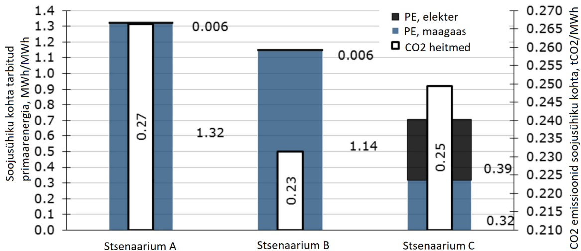
Joonis 10.7. Primaarenergia tarbimine soojuste tootmiseks ja CO 2 heitmed kolme stsenaariumi korral
