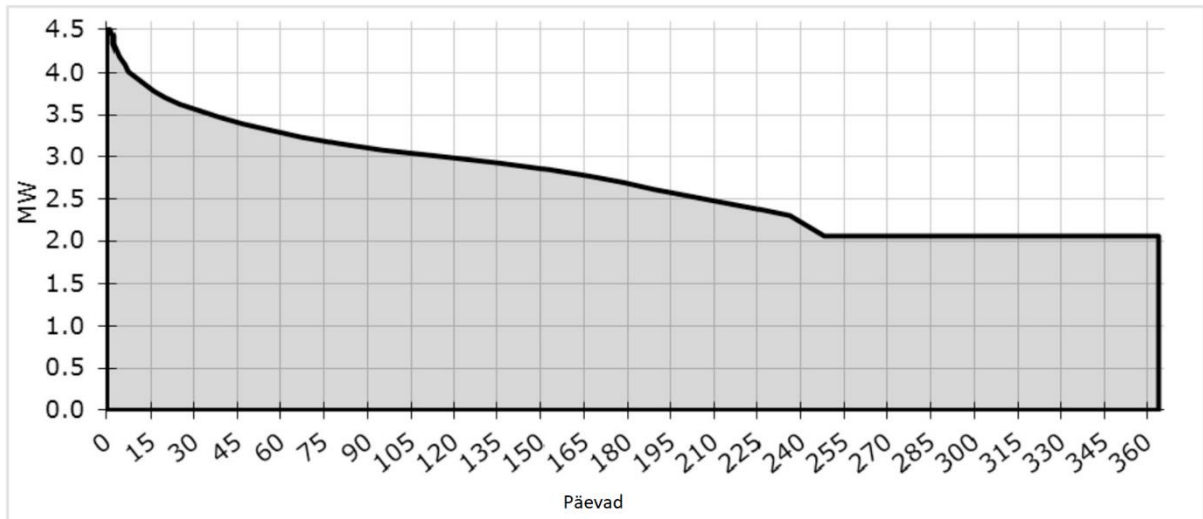
Joonis 10.4. Piirkonna soojuskoormuse graafik (stsenaarium B)
